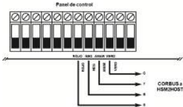
Figure 2-23 Diagrama de cableado del HSM2HOSTx
