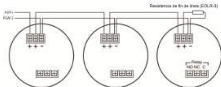
Figure 2-35 Cableado de detector de humos de dos hilos
