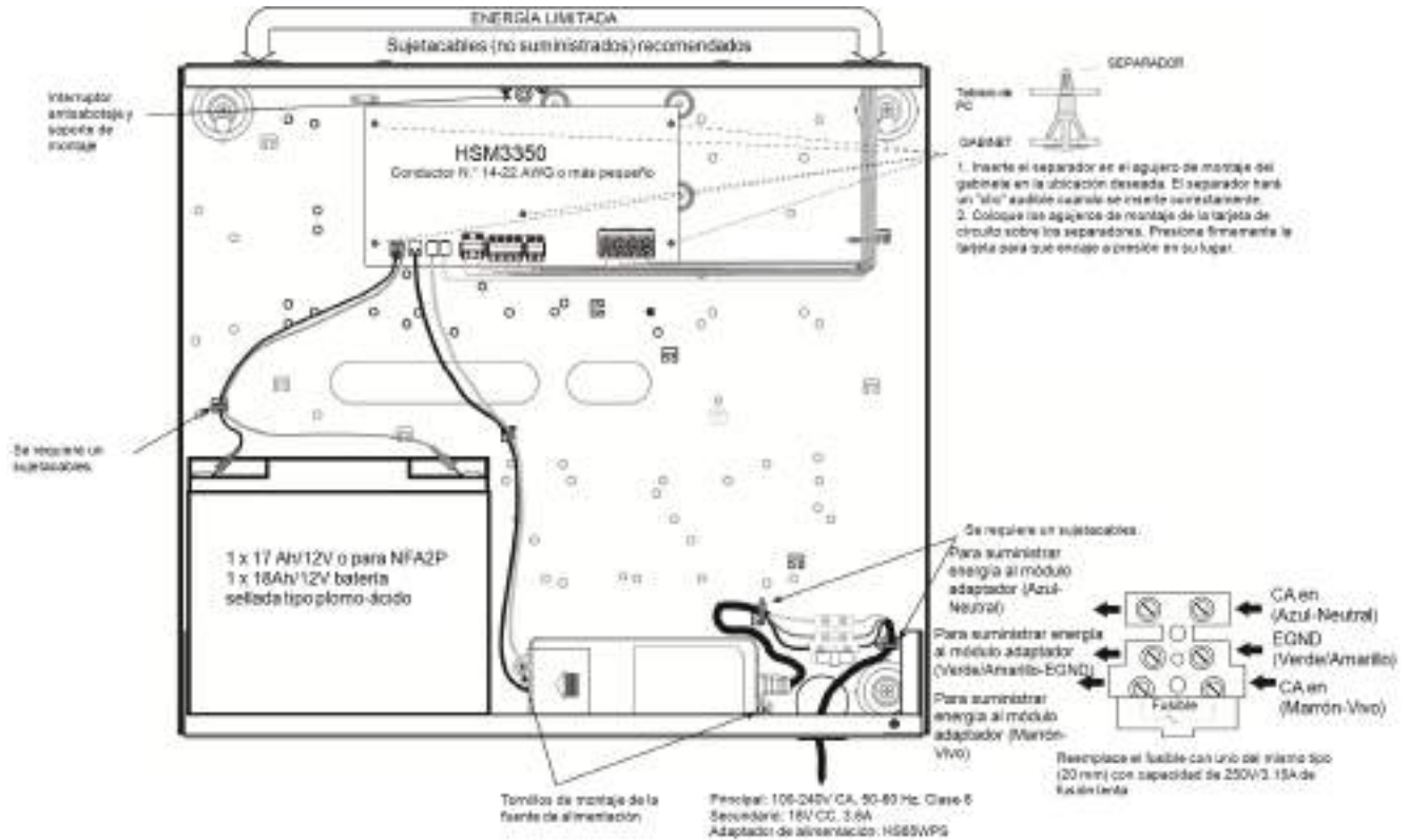
Figure 2-17 Cableado del HSM3350 para el gabinete HSC3020
