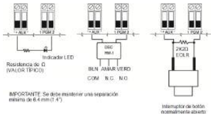
Figure 2-32 Salida LED con resistencia limitadora de corriente y salida opcional de controlador de relé.
