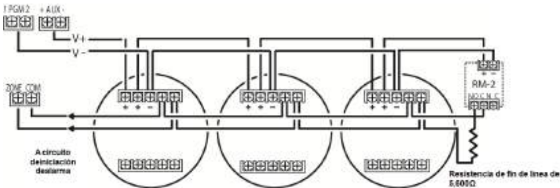
Figure 2-34 Cableado del detector de humo
