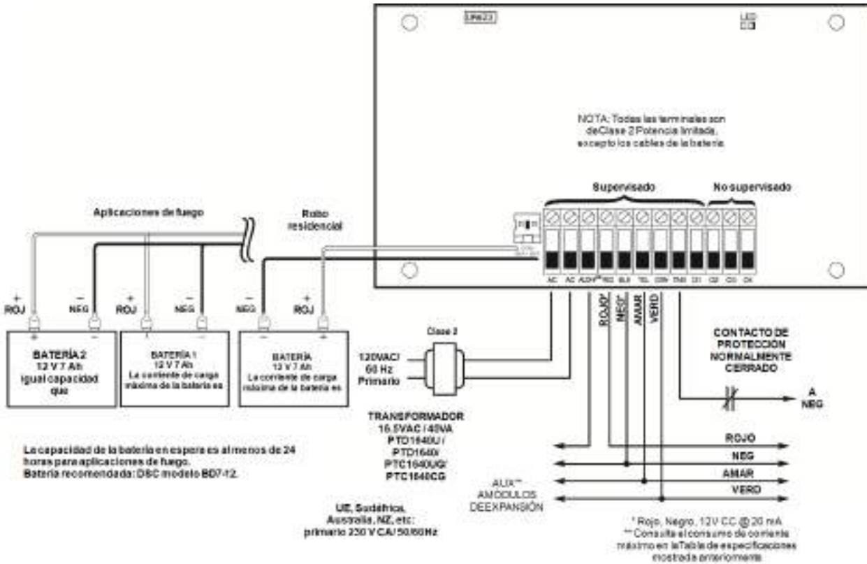
Figure 2-24 Cableado de la fuente de alimentación del HSM2300/2204
