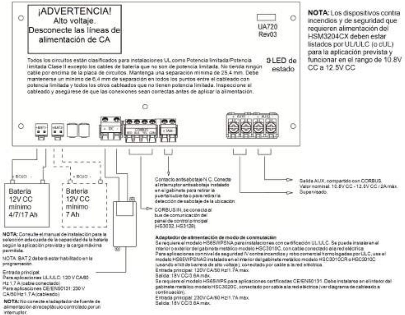
Figure 2-25 Cableado de la fuente de alimentación del HSM3350
