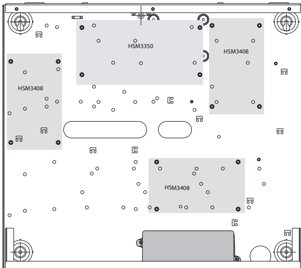
Figure 2-6 Módulos HSM3350 y HSM3408 en el gabinete HSC3020C
