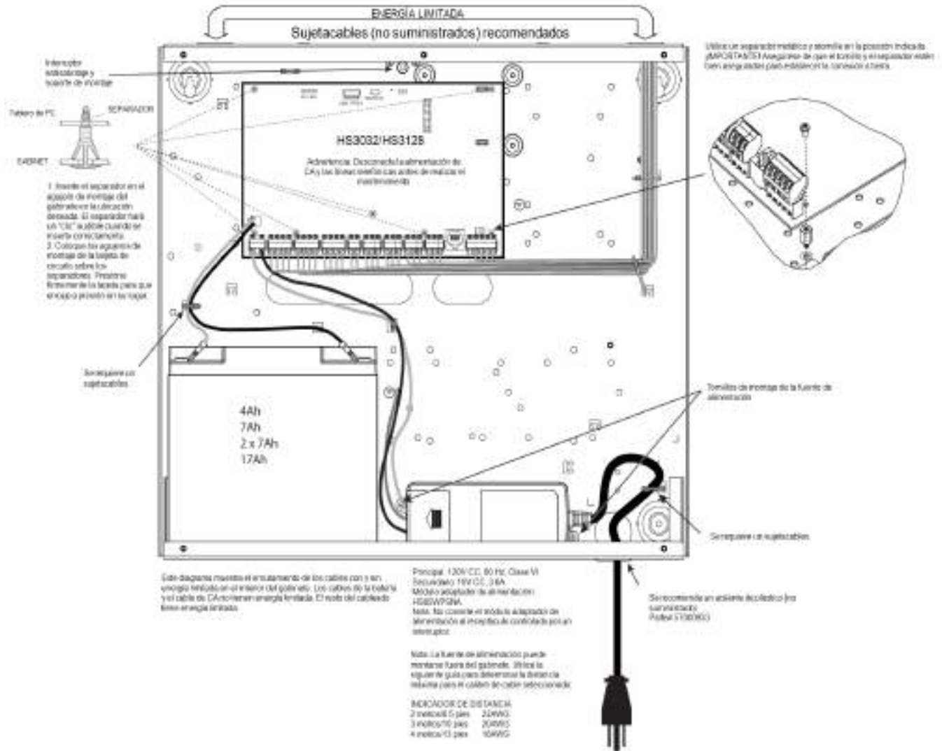
Figure 2-9 Cableado del panel para el HSC3020C (para Norteamérica)
