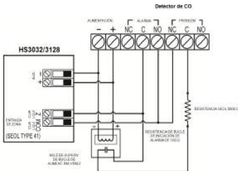
Figure 2-36 Cableado del detector de CO
