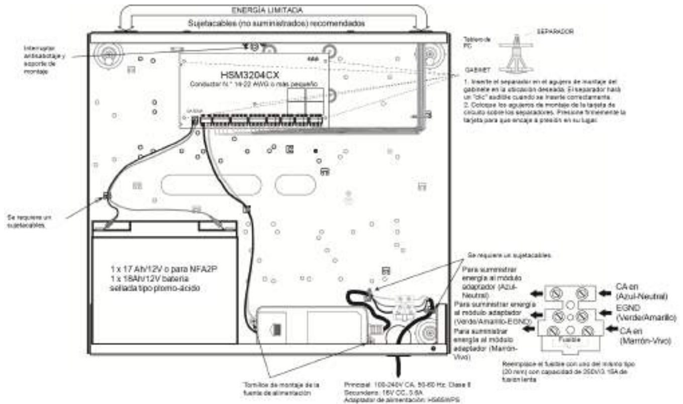
Figure 2-16 Cableado del panel para el gabinete HSC3020
