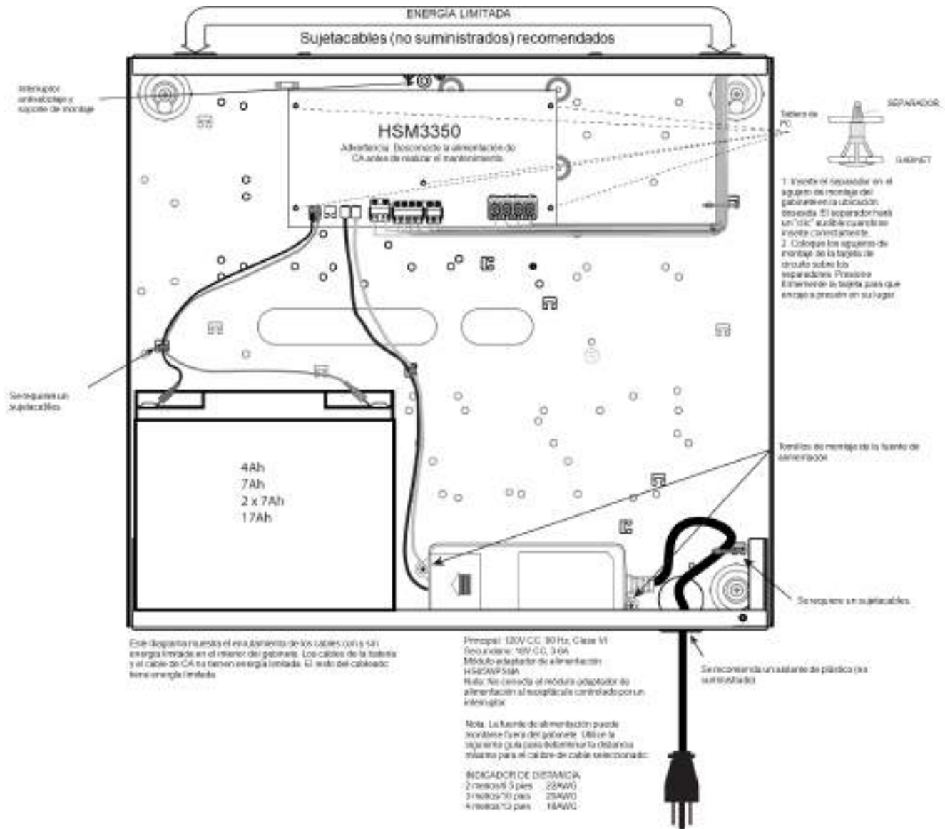
Figure 2-13 Cableado para Norteamérica del HSM3350 en el gabinete HSC3020
