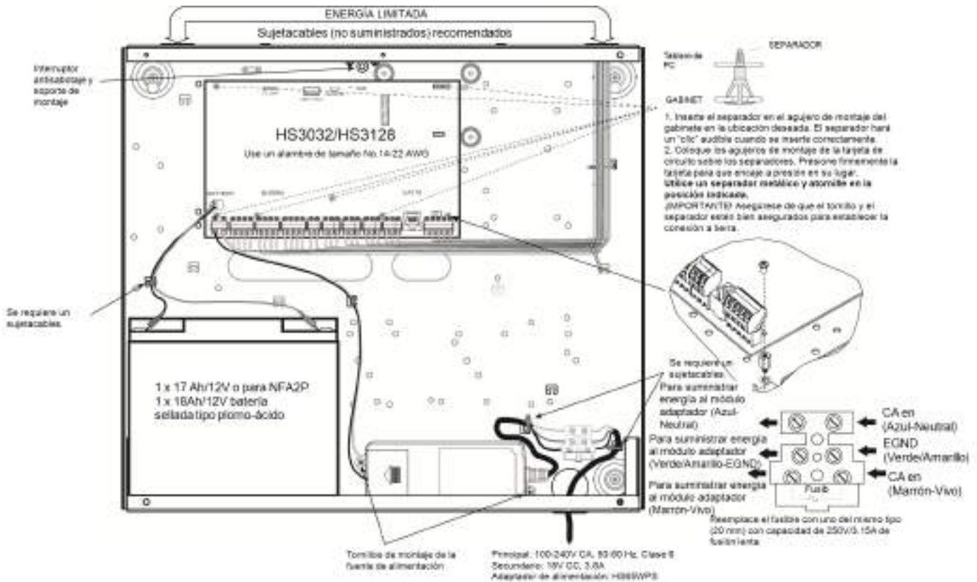
Figure 2-14 Cableado del panel para el gabinete HSC3020C
