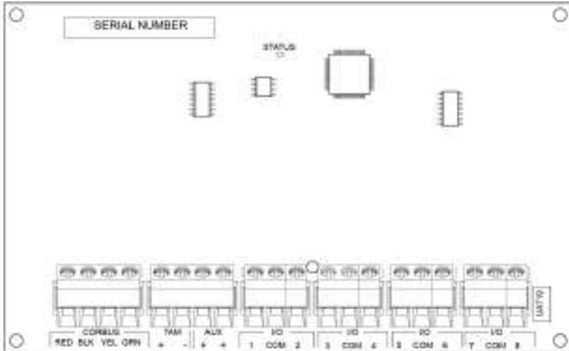
Figure 2-20 Módulo de expansión de 8 zonas HSM3408
