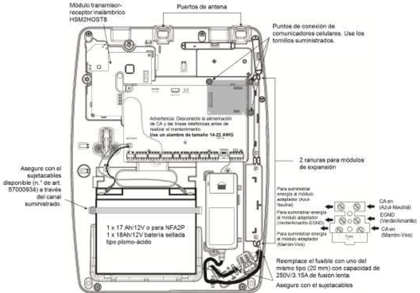
Figure 2-15 Cableado del panel para el gabinete HSC3020CP
