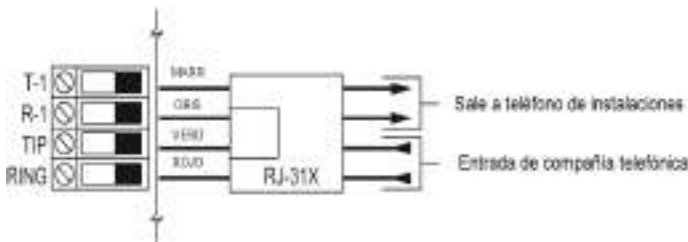
Figura 1-10 Cableado de línea telefónica
