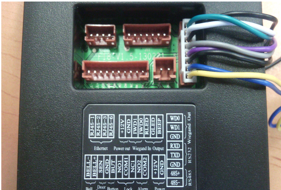
Conexion RS485 en F18
